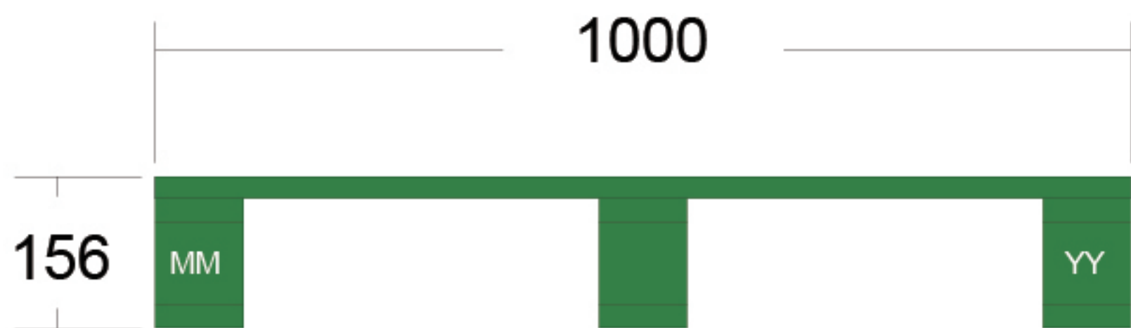
正视图
