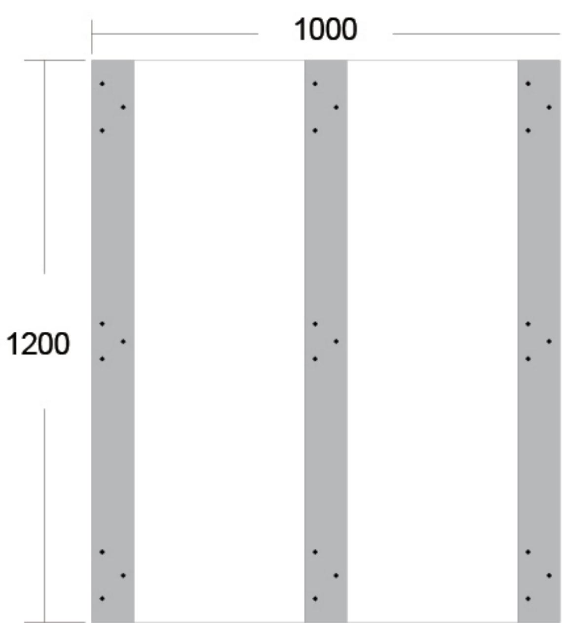
底视图
